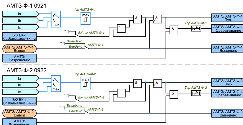
Рисунок 2.34 – Функциональная схема ступеней АМТЗ-Ф
