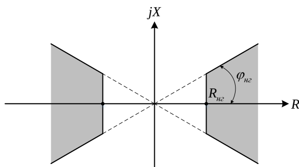
Рисунок 2.4 – Характеристика срабатывания измерительного органа отстройки от нагрузки
