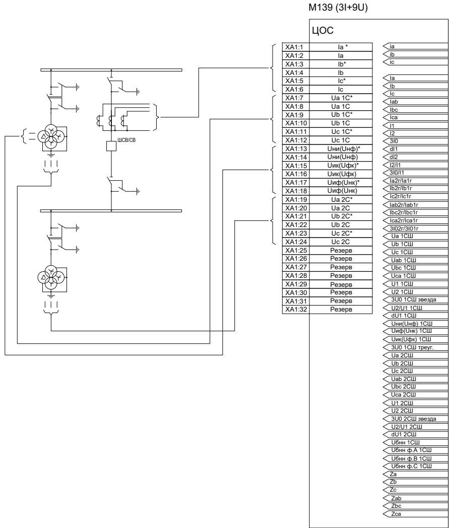
Рисунок Б.1 – Вариант подключения аналоговых цепей ТТ и ТН к устройству
